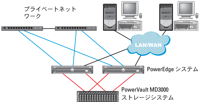
図 1-3. SAS クラスターと PowerVault MD3000 のケーブル接続
